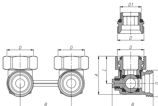
Габаритные размеры 216132
