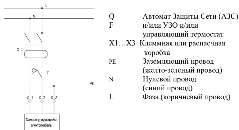
Рис. 2. Схема подключения электрообогрева кровельной воронки HL64.1 к электрической сети.
