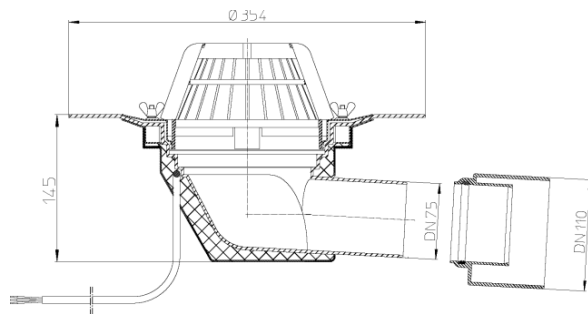
Рис. 1. Кровельная воронка HL64.1.
