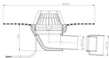
Рис. 1. Кровельная воронка HL64.1H.
