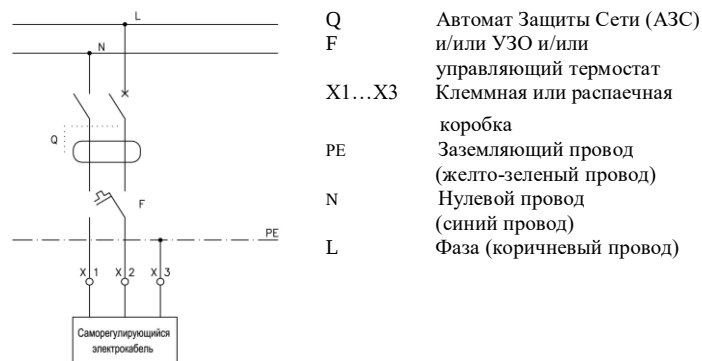
Рис. 5. Схема подключения электрообогрева кровельной воронки HL64.1H к электрической сети.
